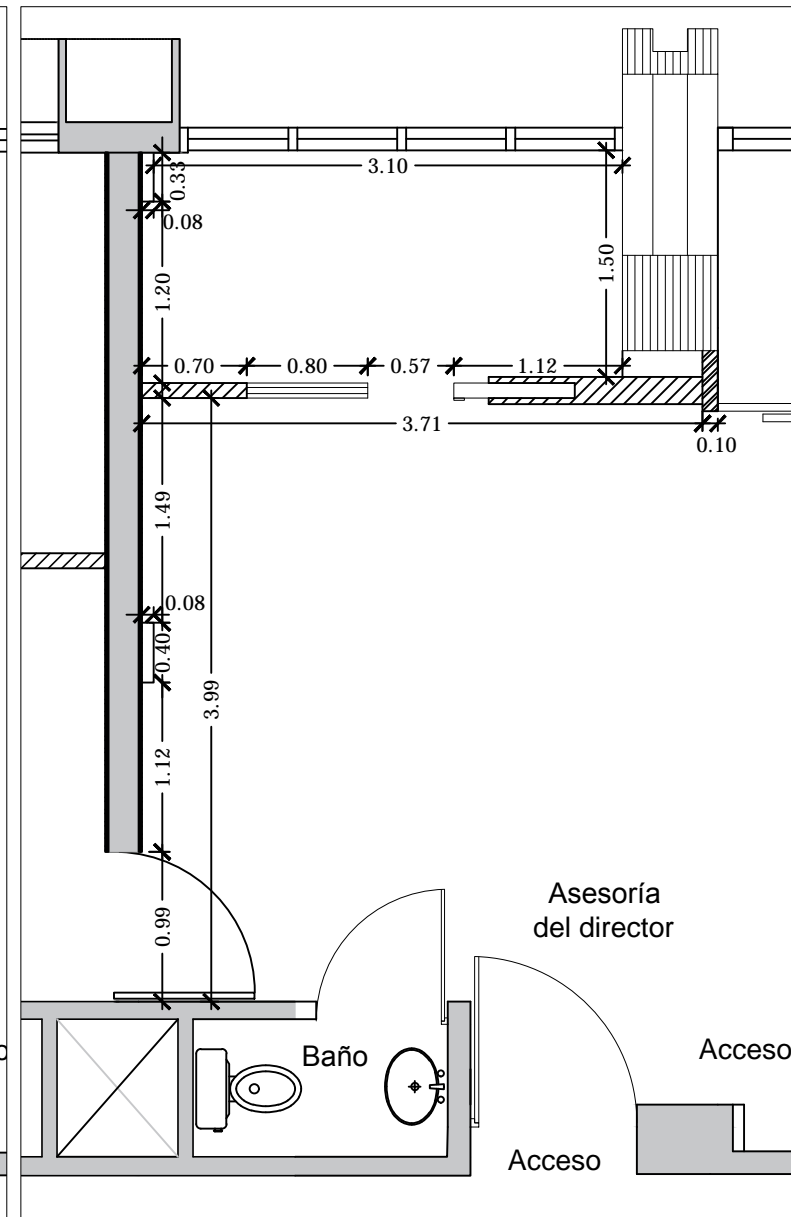
Propuesta Dimensionada 4to Nivel, Ala Sur Esc. 1:50
