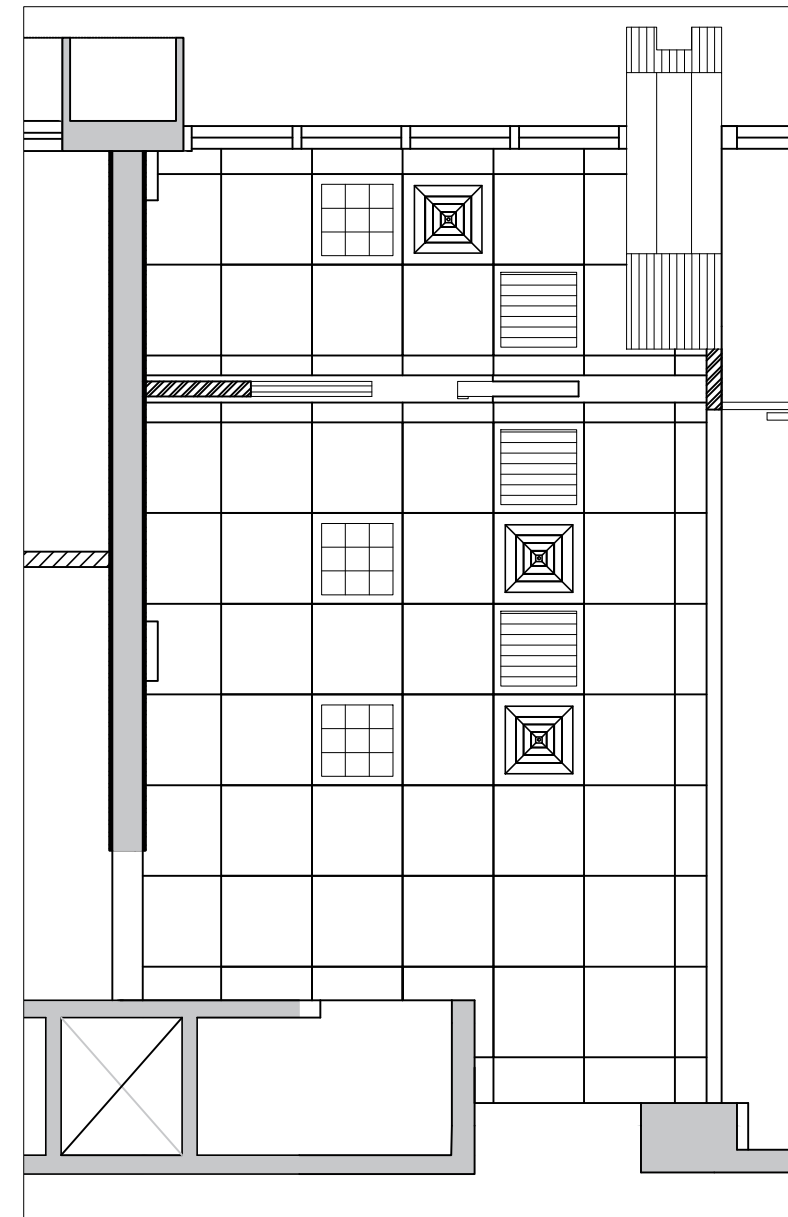
Propuesta Plafond 4to Nivel, Ala Sur Esc. 1:50
