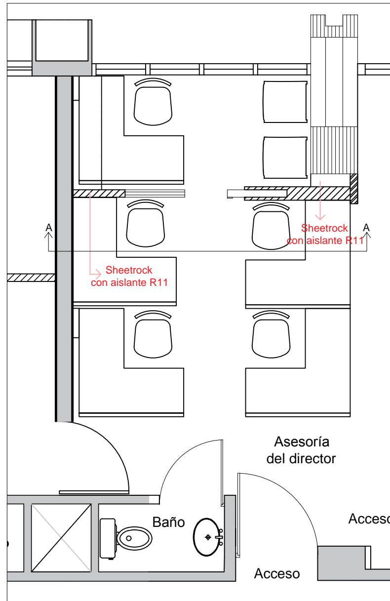
Propuesta Arquitectónica 4to Nivel, Ala Sur Esc. 1:50
